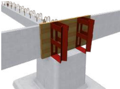
ÉQUERRES DE COFFRAGE Les équerres permettent d'assurer sans outillage spécifique le coffrage à sec des longrines.
