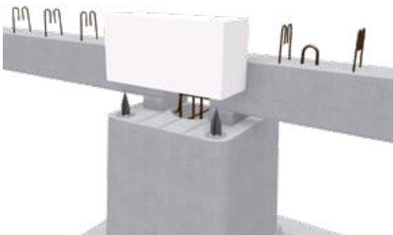
COFFRAGE PSE Mise en place simple du coffrage perdu en PSE afin d'éviter les ponts thermiques grâce aux connecteurs NEO.
