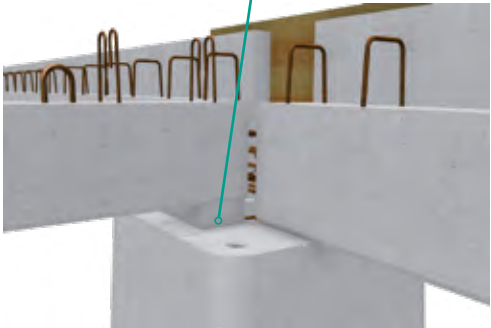
CALES BÉTON Positionnées sous la poutre, elles permettent de gérer simplement les différences de niveaux.
