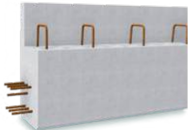
Poutre PCS
